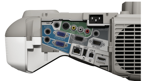
Interfaz EB-485W
