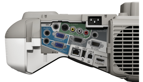
Interfaz EB-480
